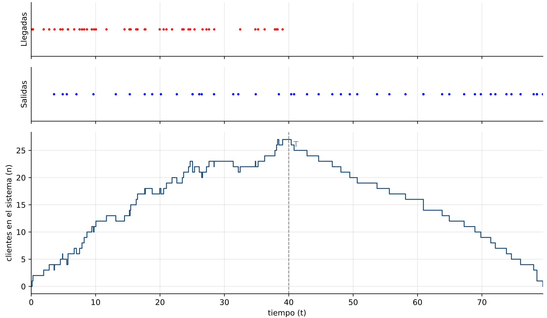
Escenario B: llegadas \text{Exp}(\lambda=1) , servicio N(2, 1) truncada en 0, T = 40
